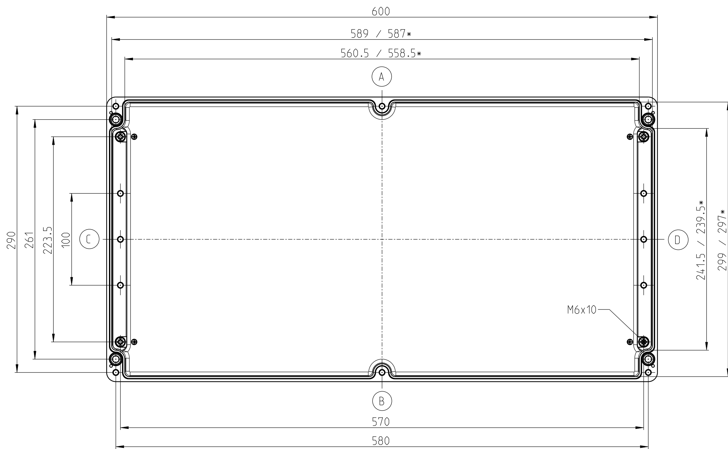
UNTERTEIL
