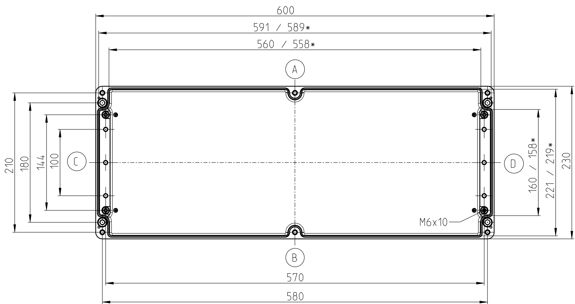
UNTERTEIL
