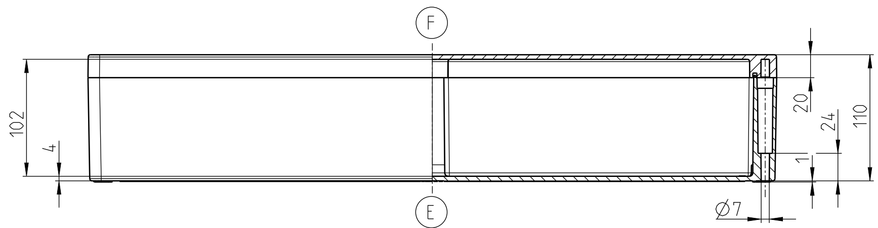
UNTERTEIL
