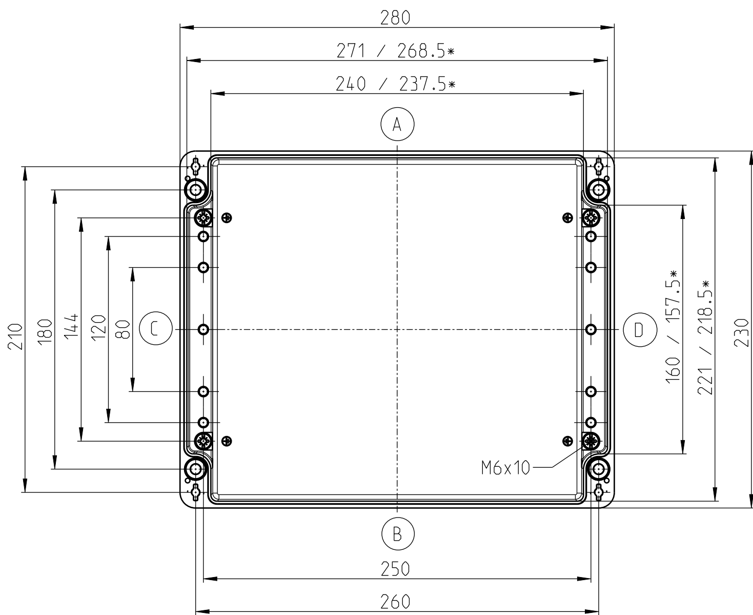
UNTERTEIL
