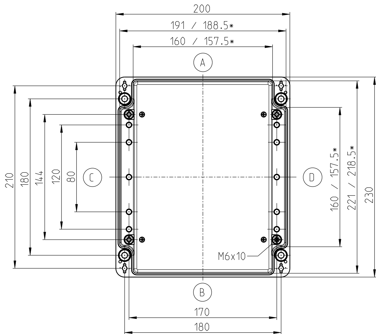
UNTERTEIL
