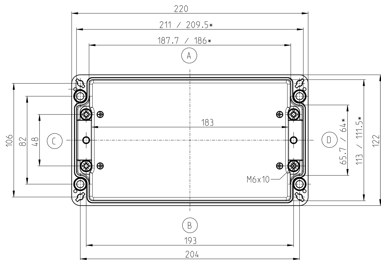
UNTERTEIL
