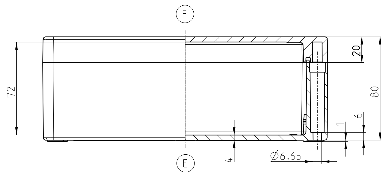
UNTERTEIL
