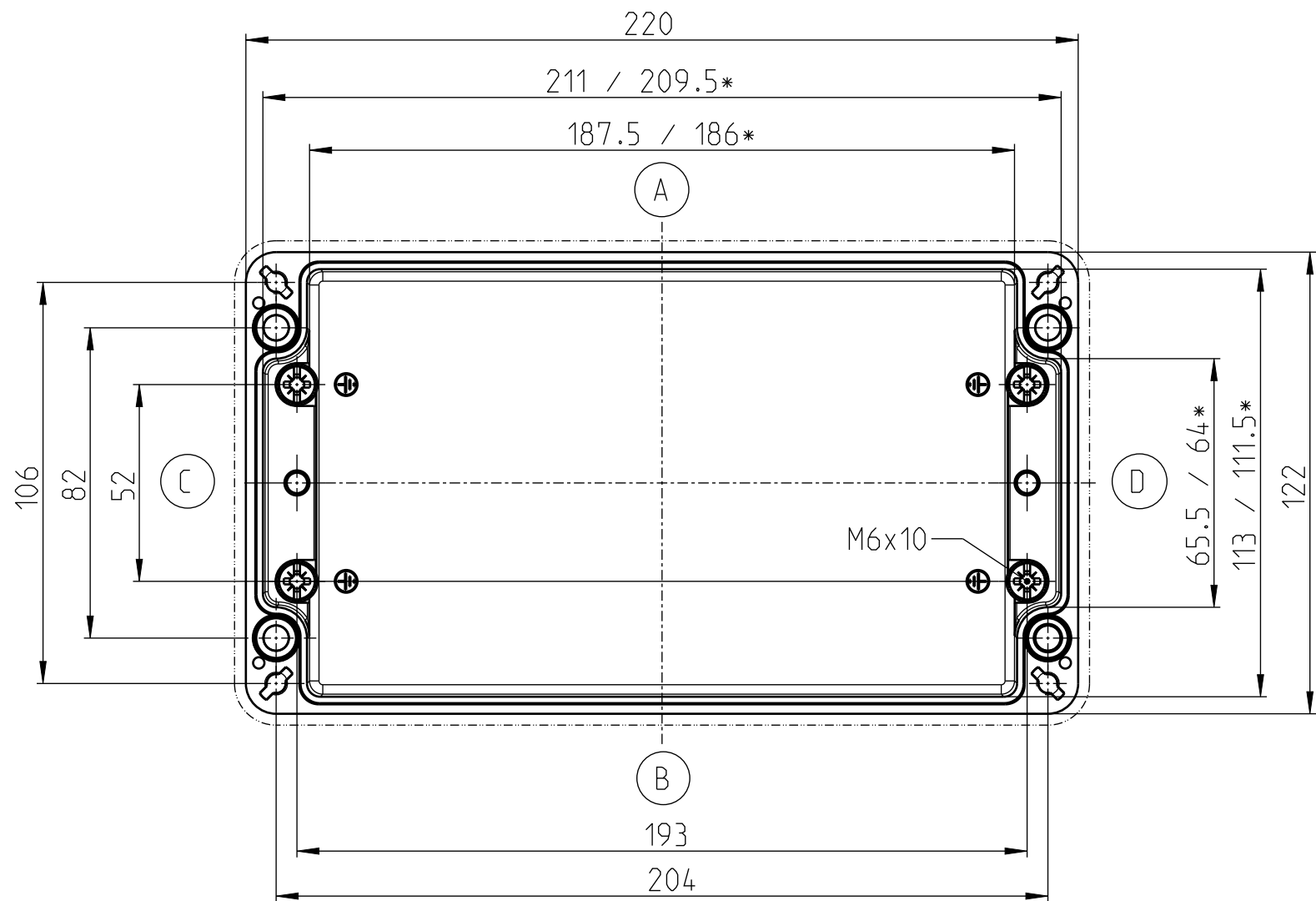
UNTERTEIL
