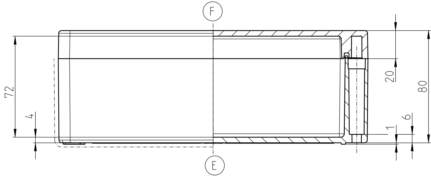
UNTERTEIL
