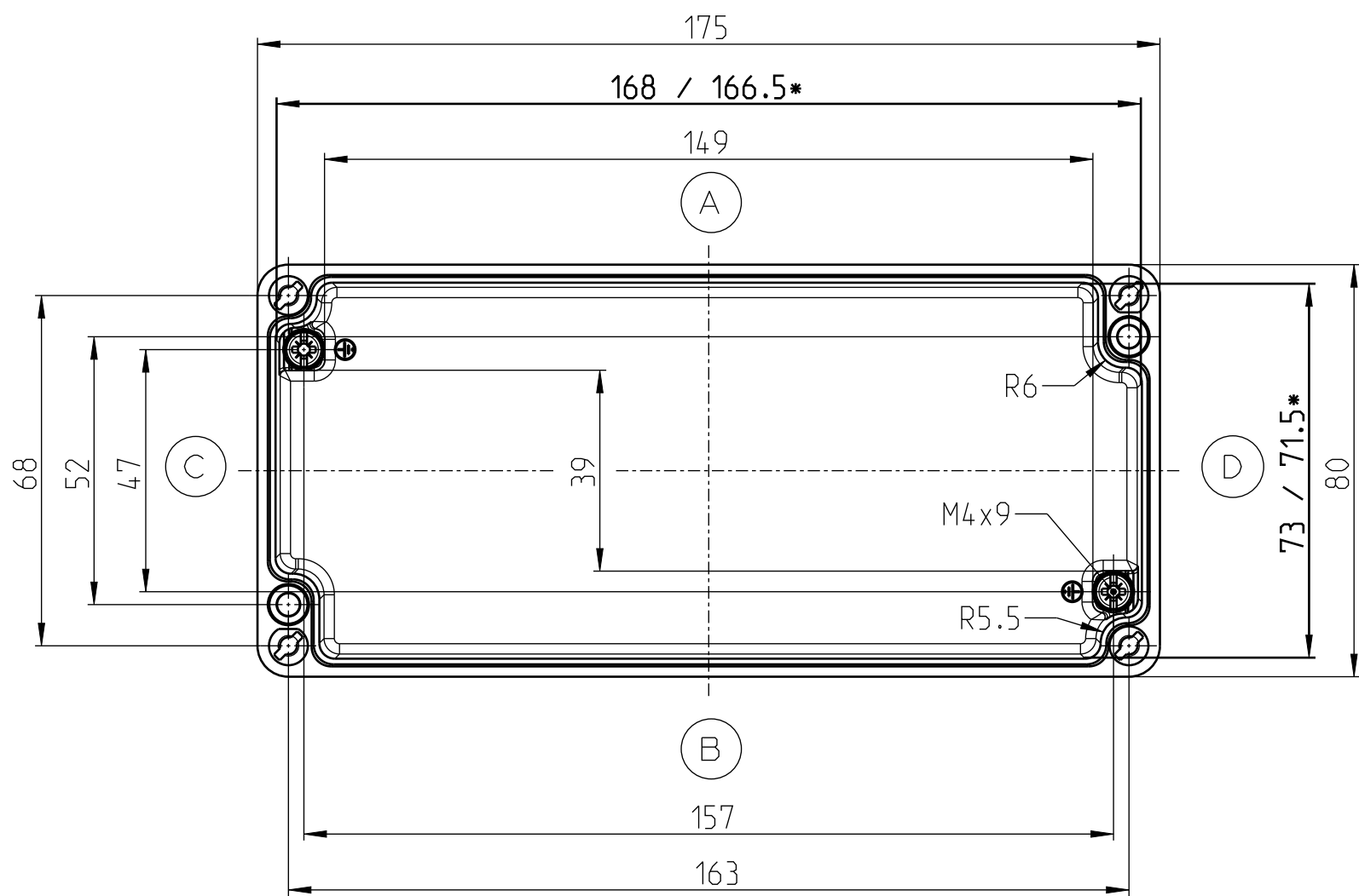
UNTERTEIL
