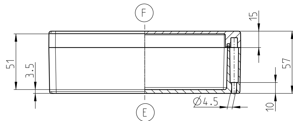
UNTERTEIL
