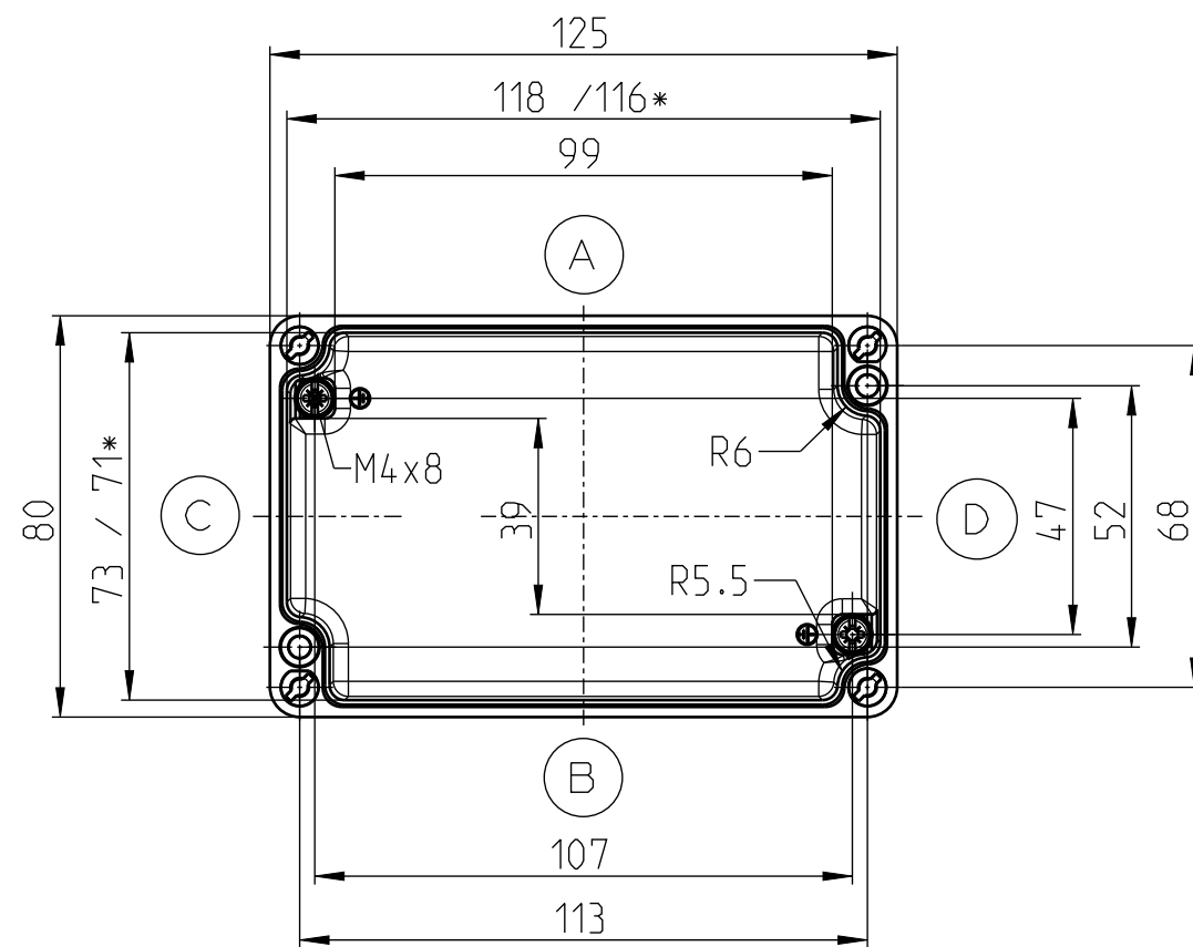
UNTERTEIL
