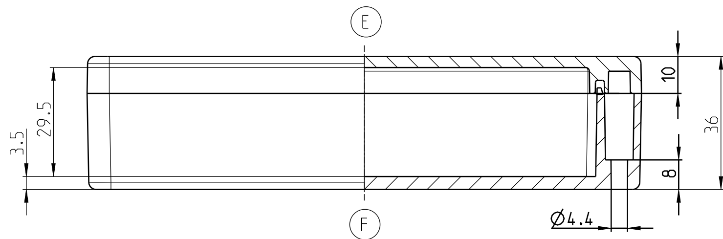
UNTERTEIL
