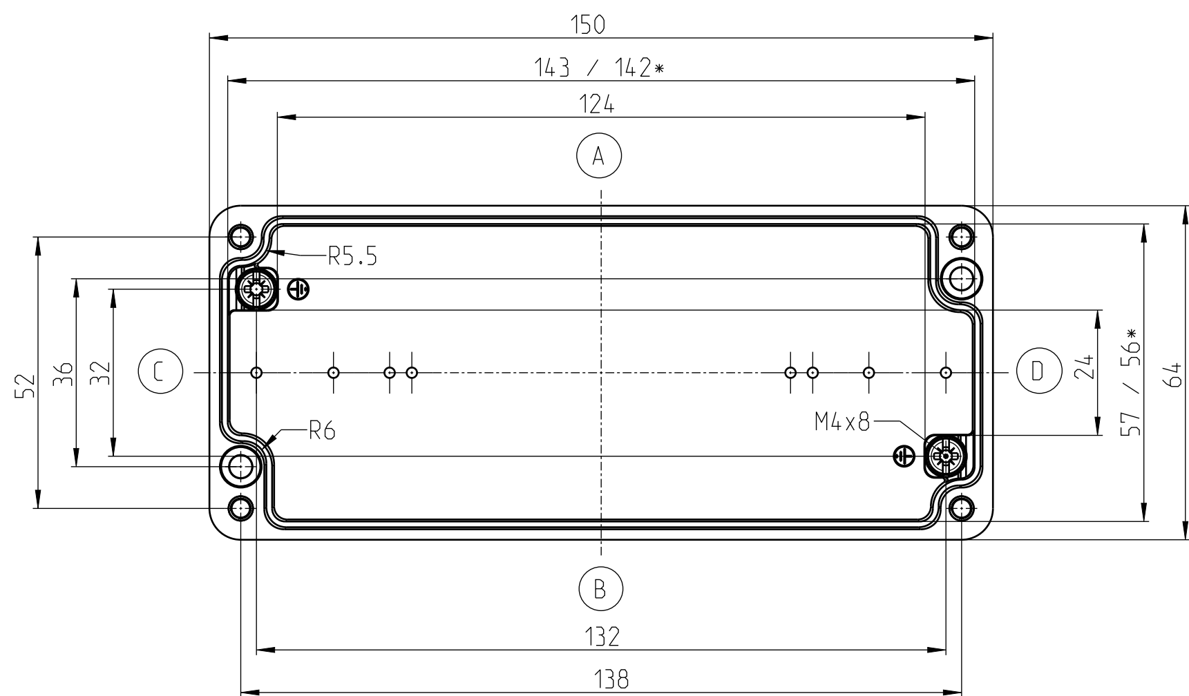
UNTERTEIL
