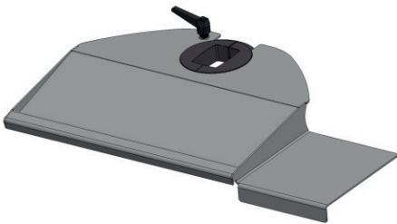
ERGO.SLIDE2 Blechablage Art.-Nr.:9806000113 RAL 9006
