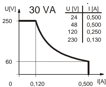
Leistungsdiagramm
