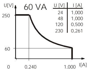
Leistungsdiagramm
