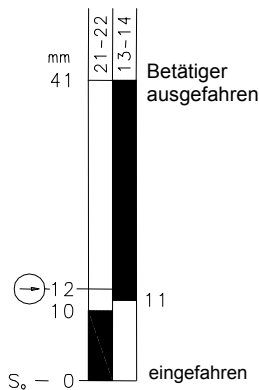
Schaltprogramm
